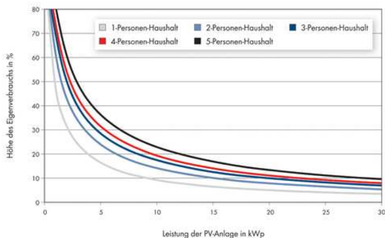
Abb. 2: Die „natürliche“ Eigenverbrauchsquote hängt ab von der Anlagenleistung und der Personenzahl im Haushalt
