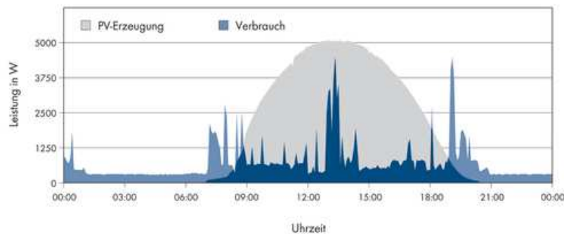
Abb. 1: Erzeugung, Verbrauch und Eigenverbrauch an einem wolkenlosen Sommertag (Vier-Personen-Haushalt und Solarstrom-Anlage mit 5 kW Peakleistung)
